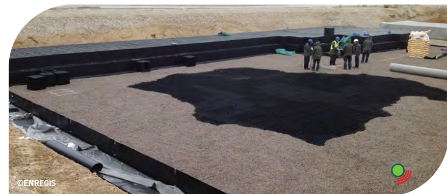
Befüllung der Behandlungsstufe einer Rigole für die Abläufe eines Asphaltwerkes mit ENREGIS/Vivo Biocalith® MR-F1 (DK)
